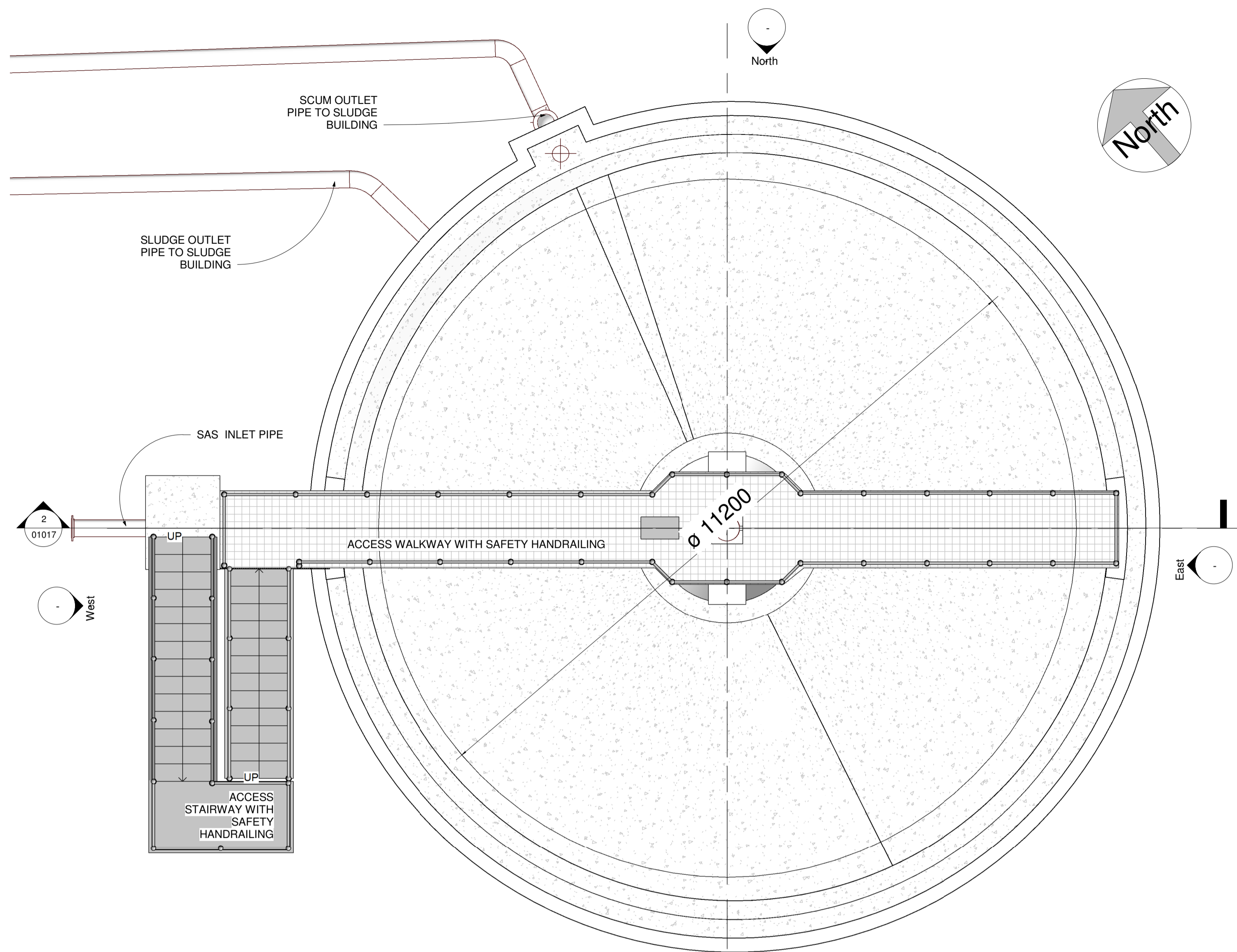
1 PFT - PLAN 1 : 50
