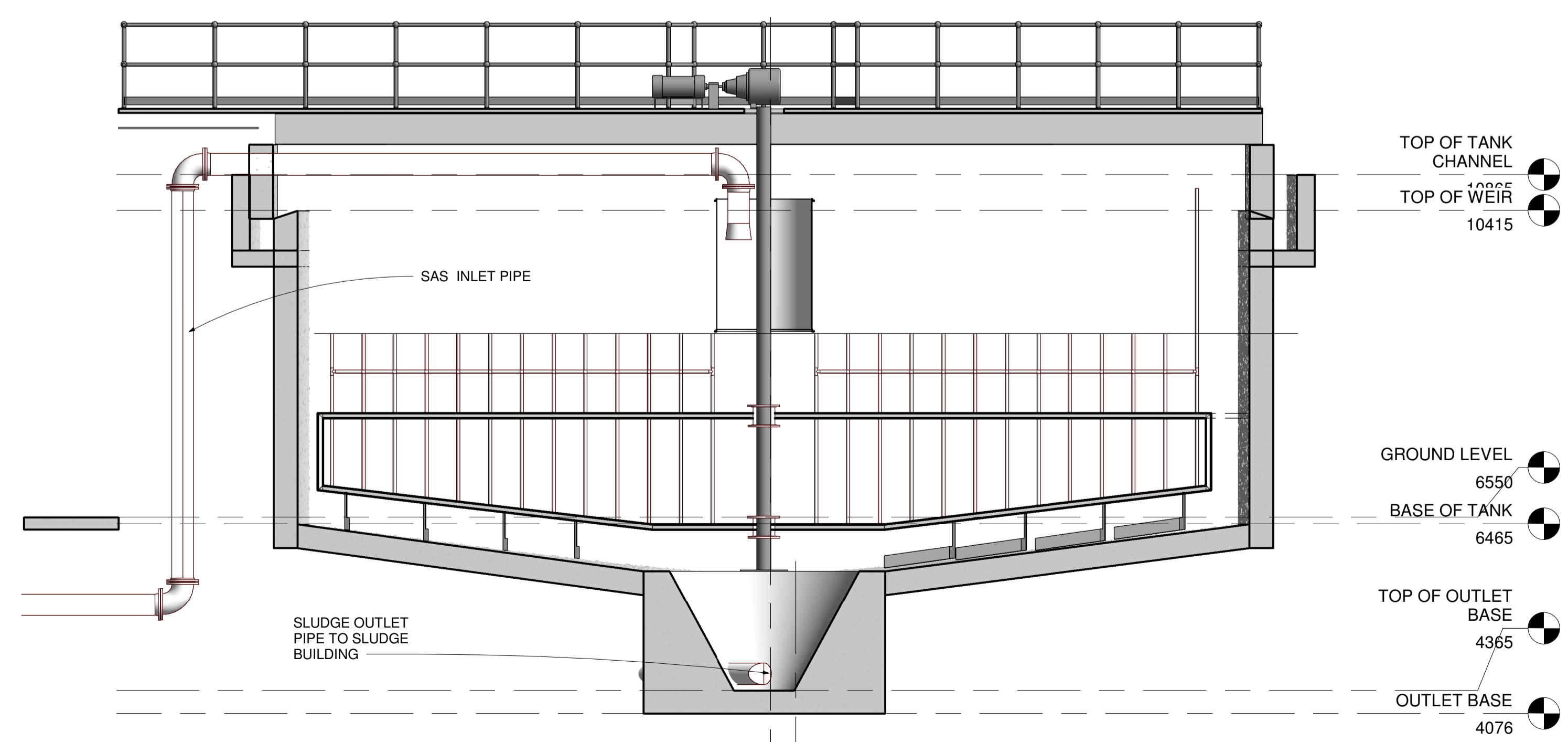
2 Section 1 1 : 50
